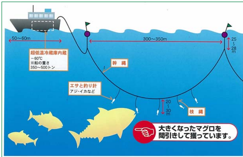
はえ縄漁業の図解
